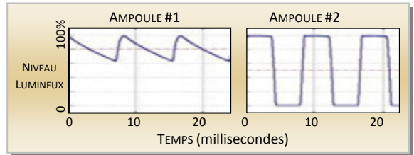
Émissions lumineuses d'ampoules DEL typiques, indiquant de hauts niveaux de scintillement
